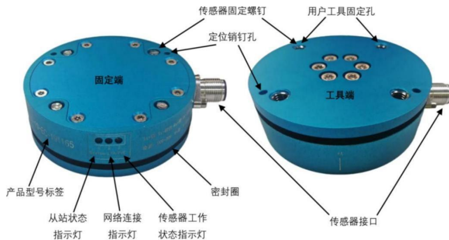
图 2.2 传感器外观结构
